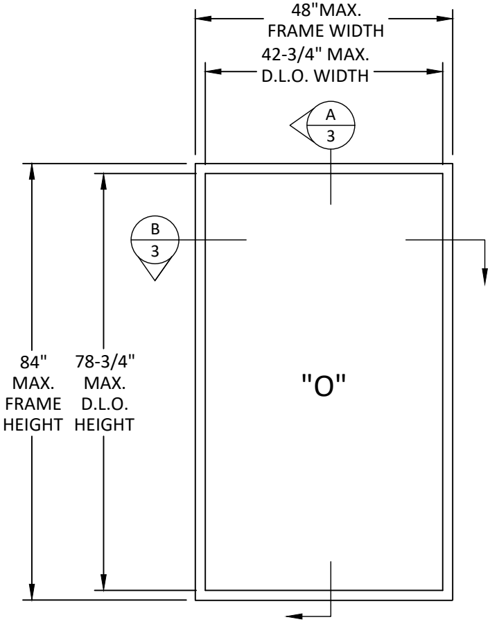
ELEVATION
