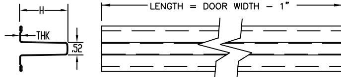
13 411186 & 412619, HEMMED STRUT
