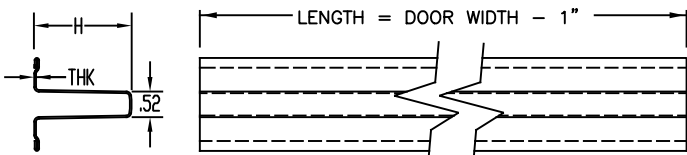
14 411186 & 412619, HEMMED STRUT
