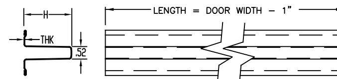
14 411186 & 412619, HEMMED STRUT
