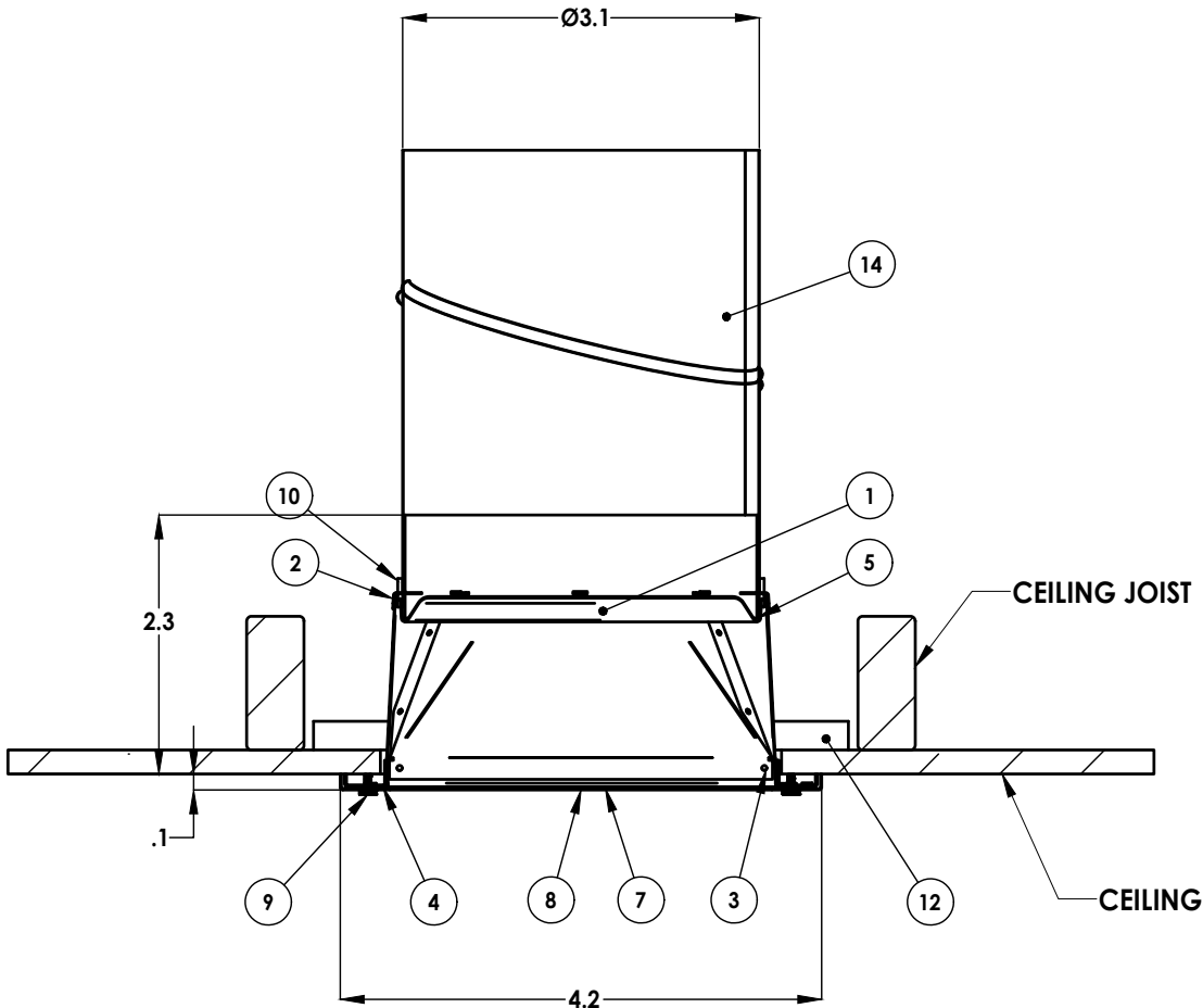
SECTION D-D
