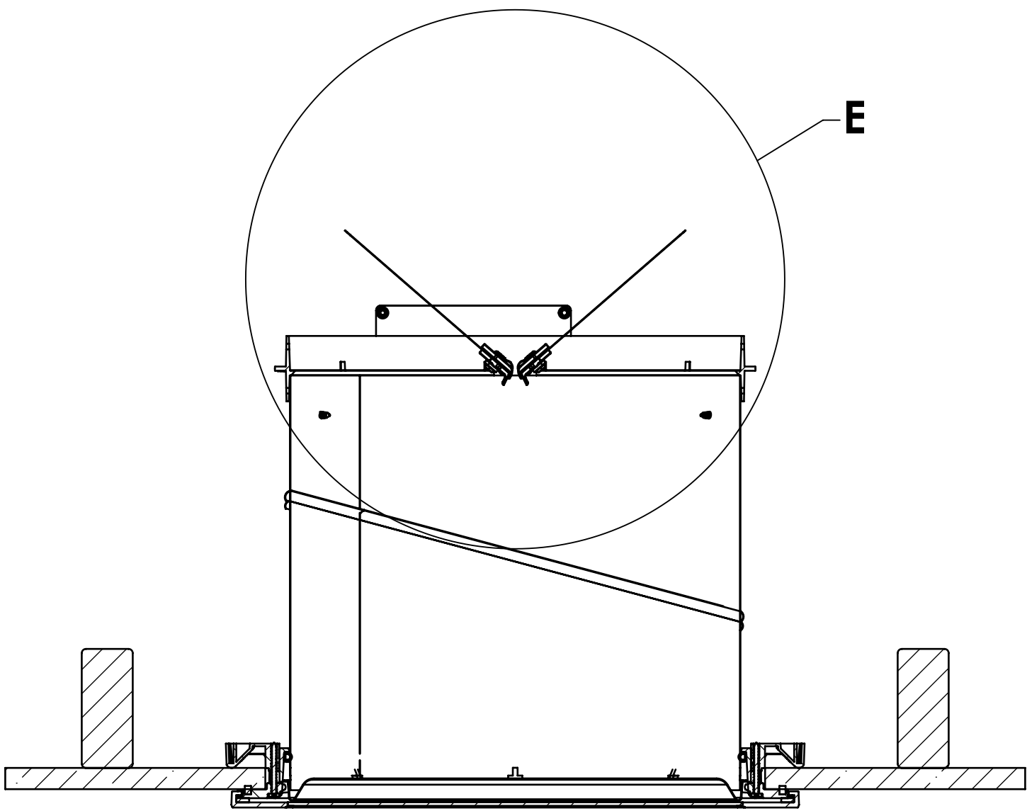
SECTION D-D
