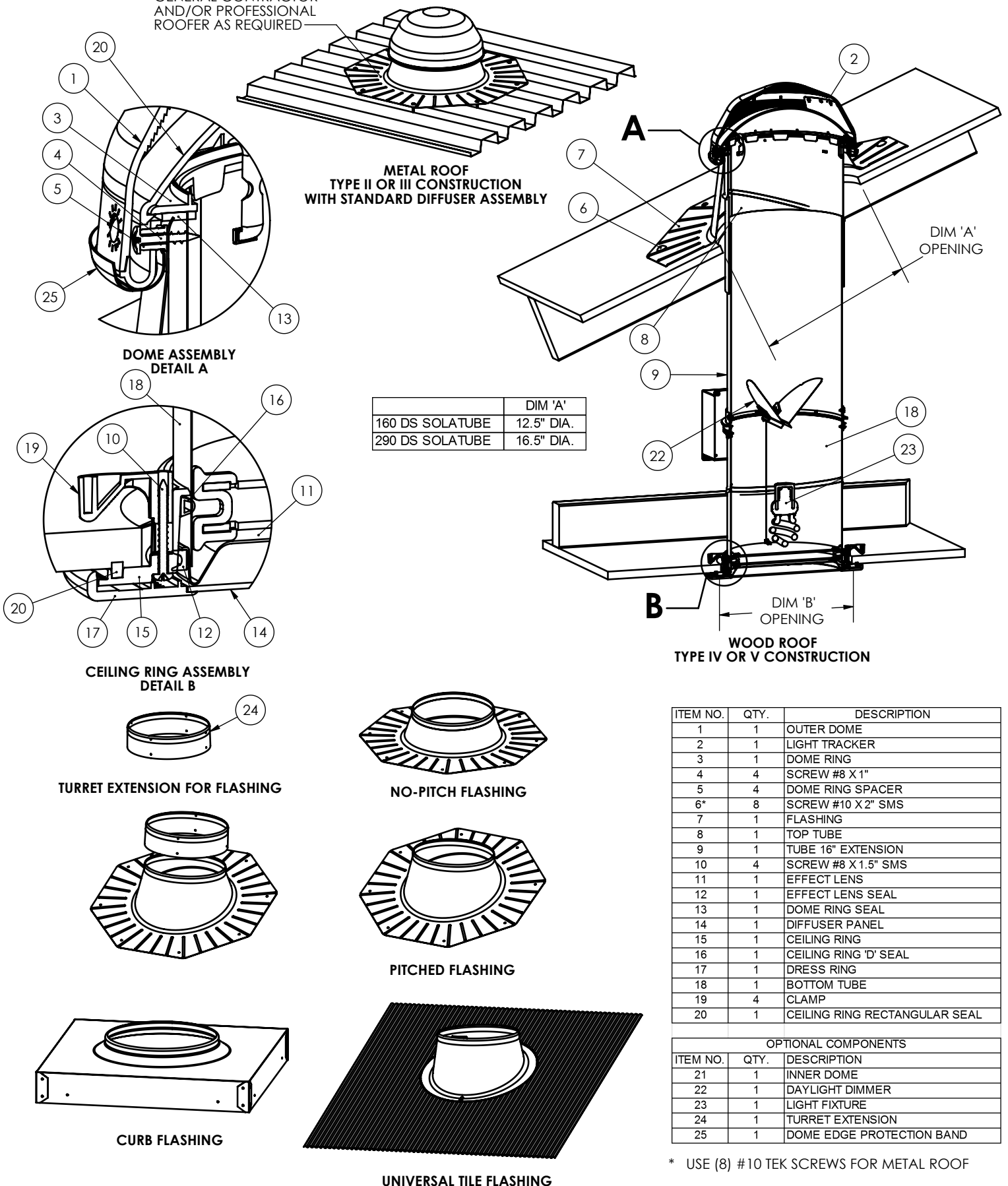
FIGURE 1 - 160 DS & 290 DS SOLATUBE WITH DETAILS
