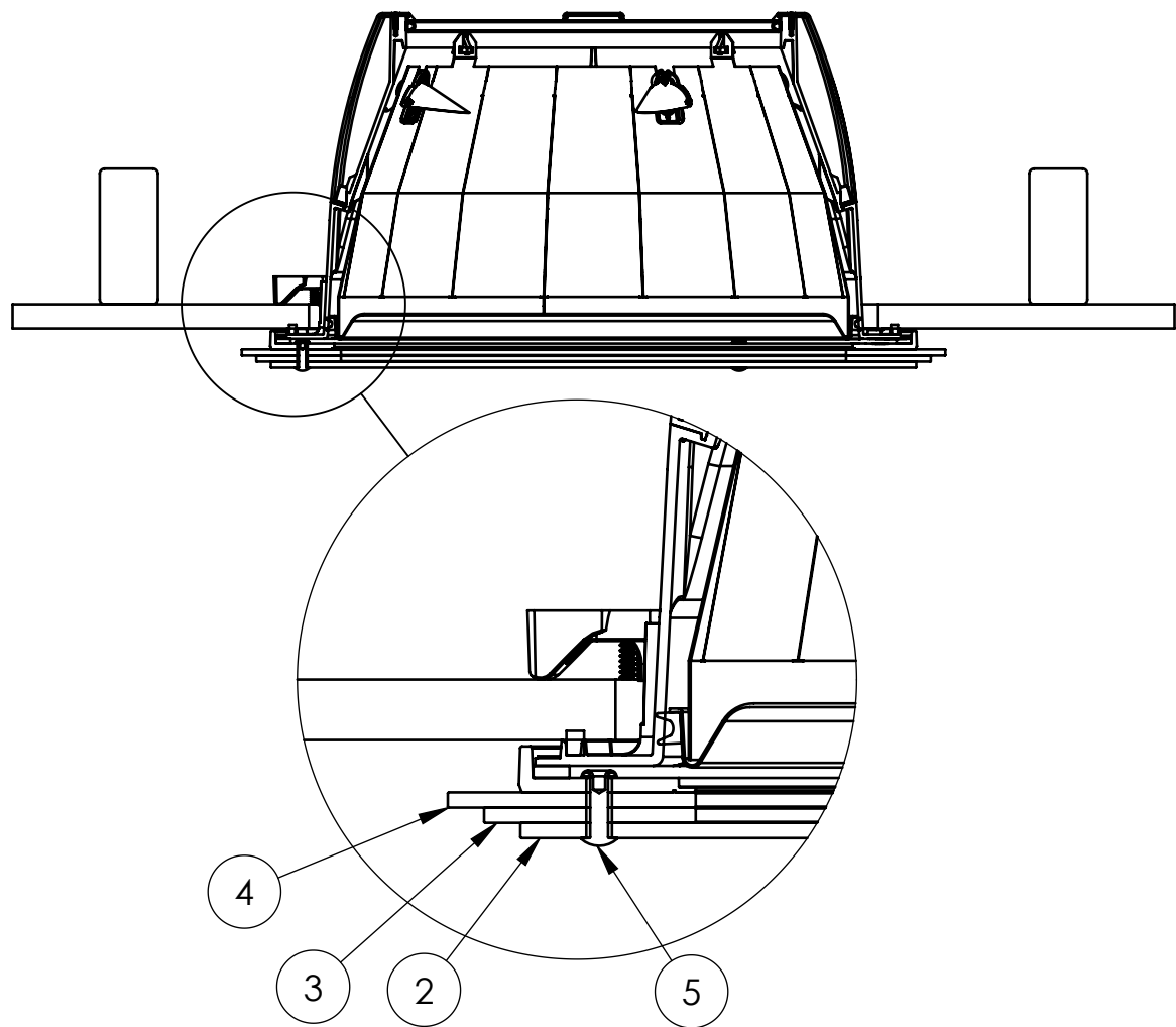
'TIER DROP' DIFFUSER ASSEMBLY
