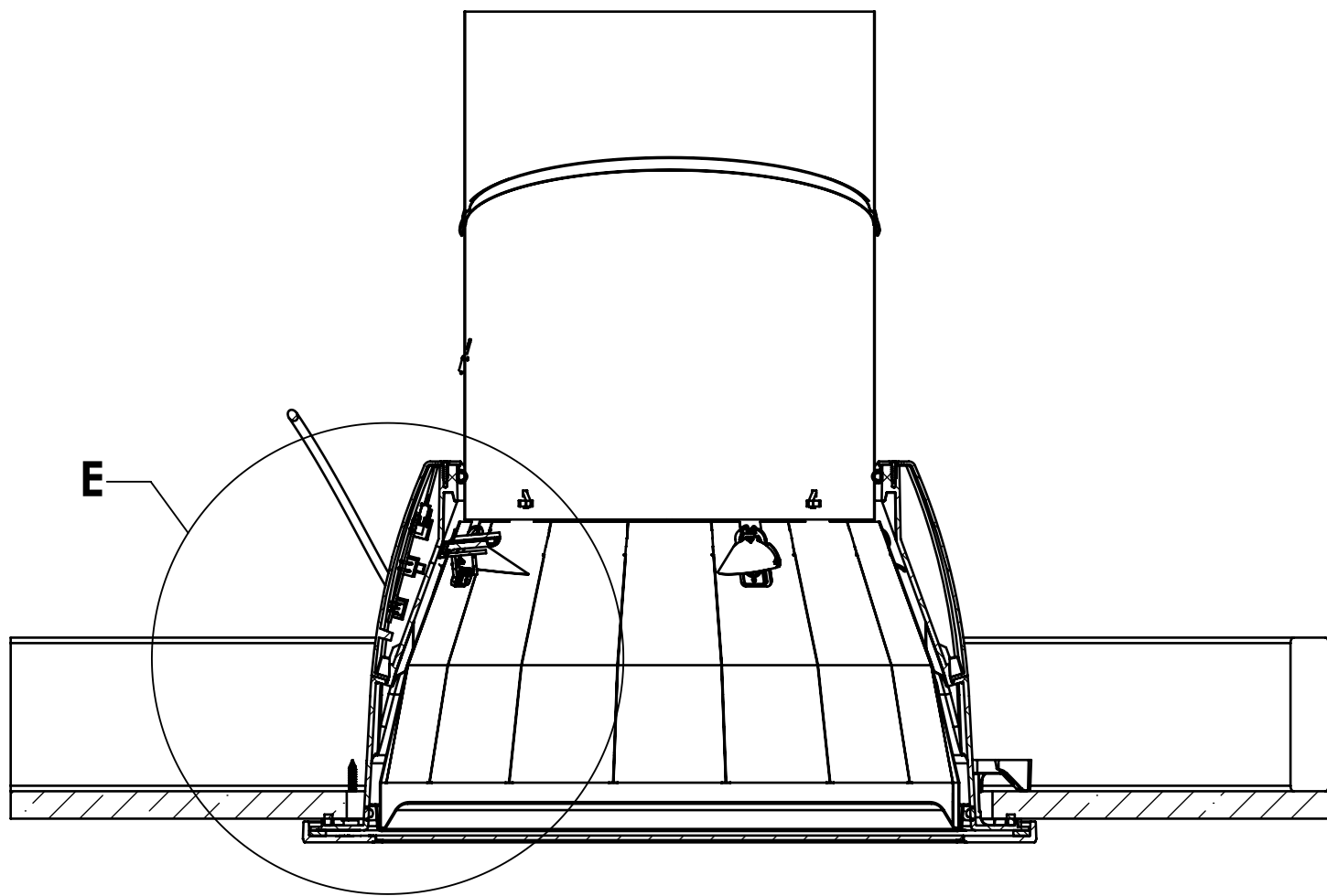
SECTION D-D
