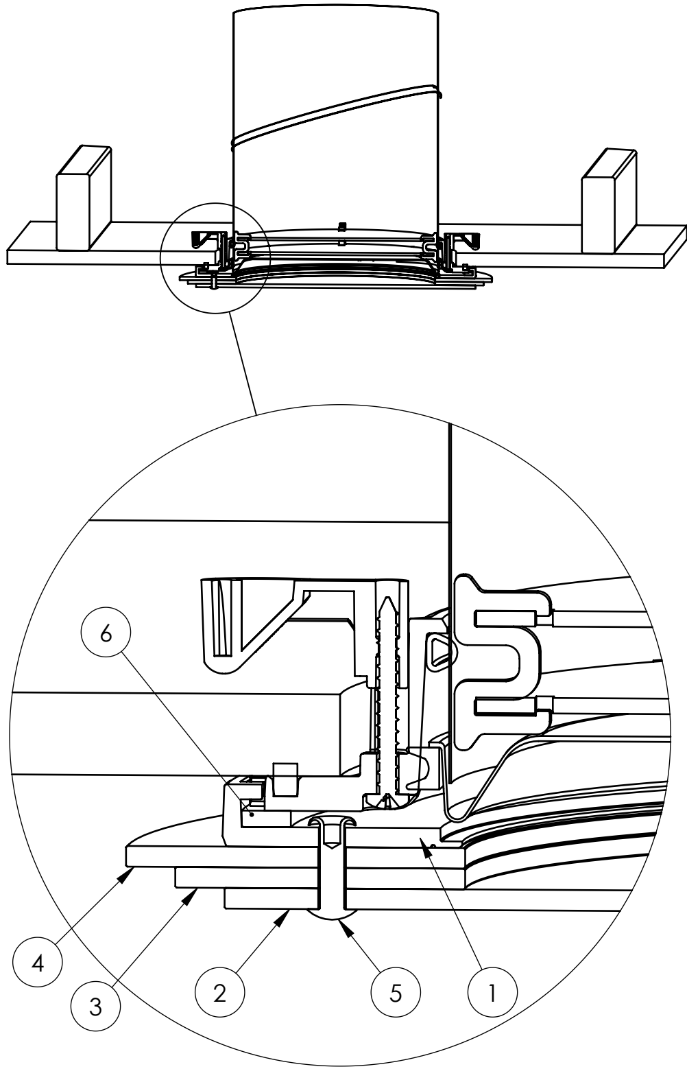
'TIER DROP' DIFFUSER ASSEMBLY
