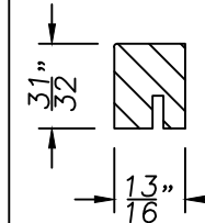
JAMB STOP (25)
