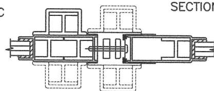
ASTRAGAL
