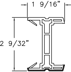
ASTRAGAL STRIP RIGID PVC
