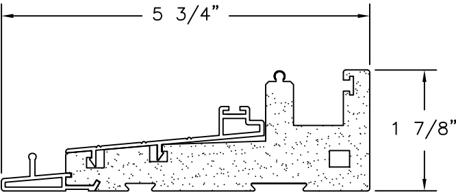
DOOR SILL
