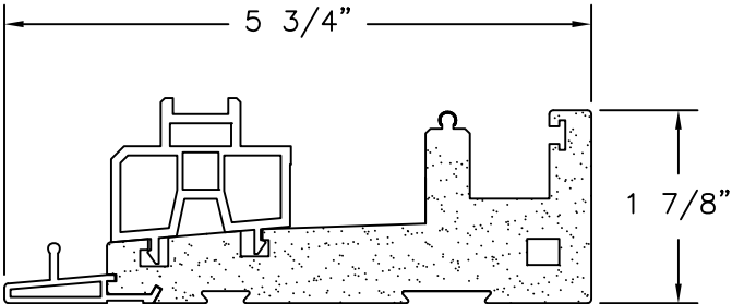
DOOR SILL
