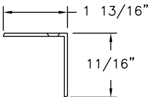
21 CORNER KEY DIE CAST
