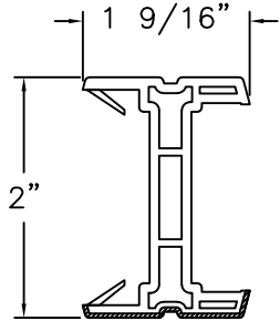
ASTRAGAL STRIP RIGID PVC
