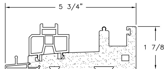
DOOR SILL
