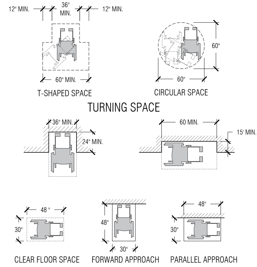
A MINIMUM CLEAR FLOOR SPACE N.T.S.
