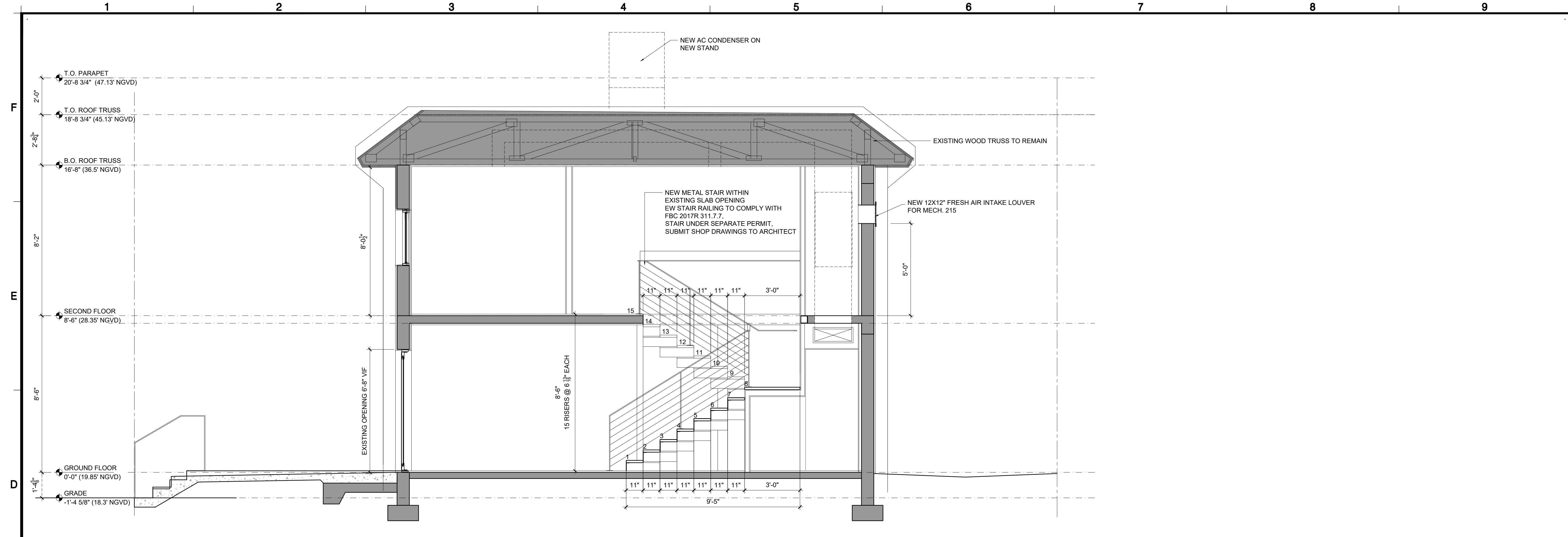
1 SECTION A-A SCALE: 3/8" = 1'-0"
