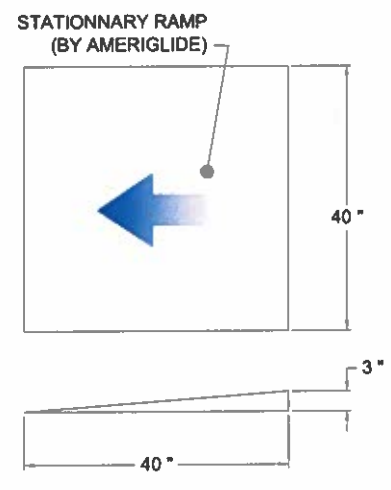
9 STATIONNARY RAMP
