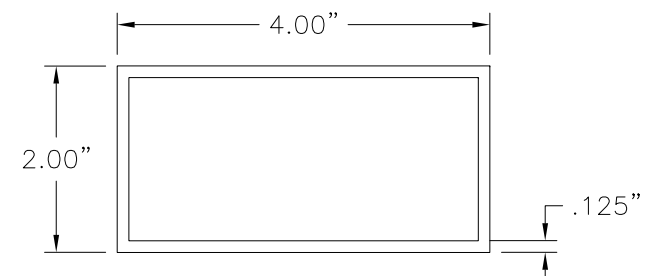
15 HEADER 6063-T5 ALUMINUM
