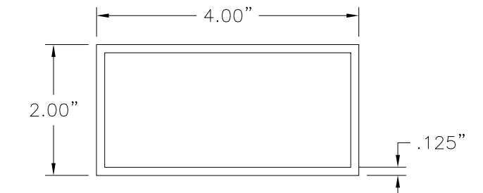
17 STORM BAR 6063-T5 ALUMINUM
