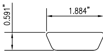
6 ASTRAGAL Scale: 1/2 FULL SIZE
