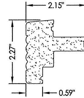
11 EXTERIOR LITEFRAME DOOR
