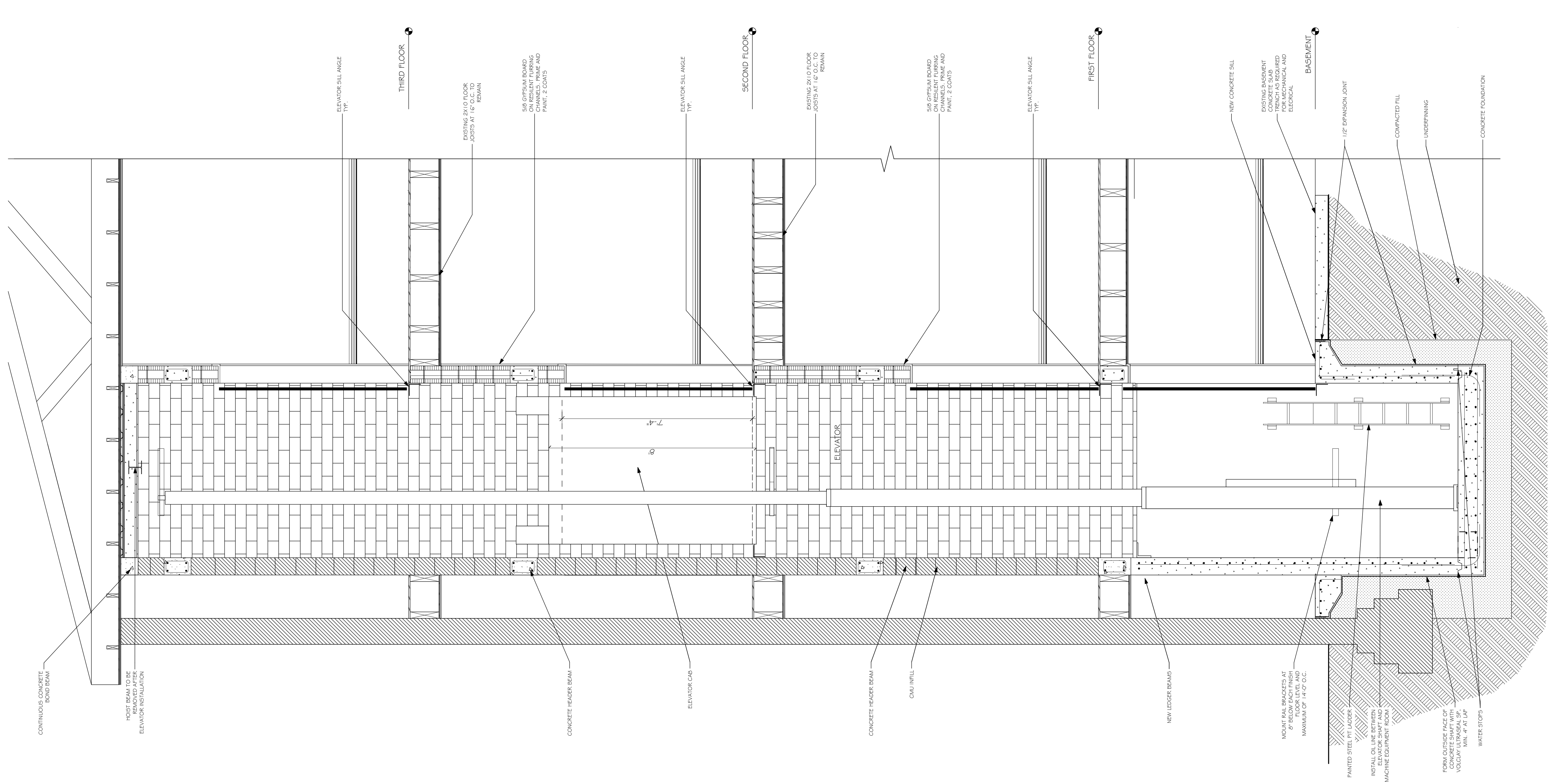
1 ELEVATOR SECTION ASI 1.2 SCALE: 1/2" = 1'-0"
